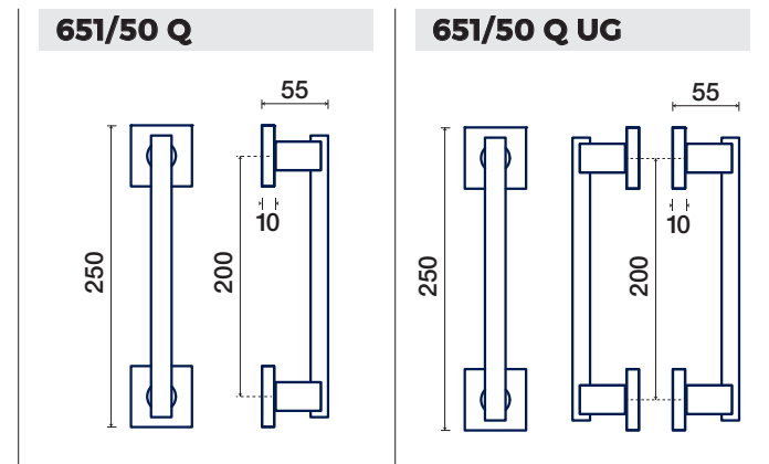
maniglie - vedi pag. 120 handles - see page 120
